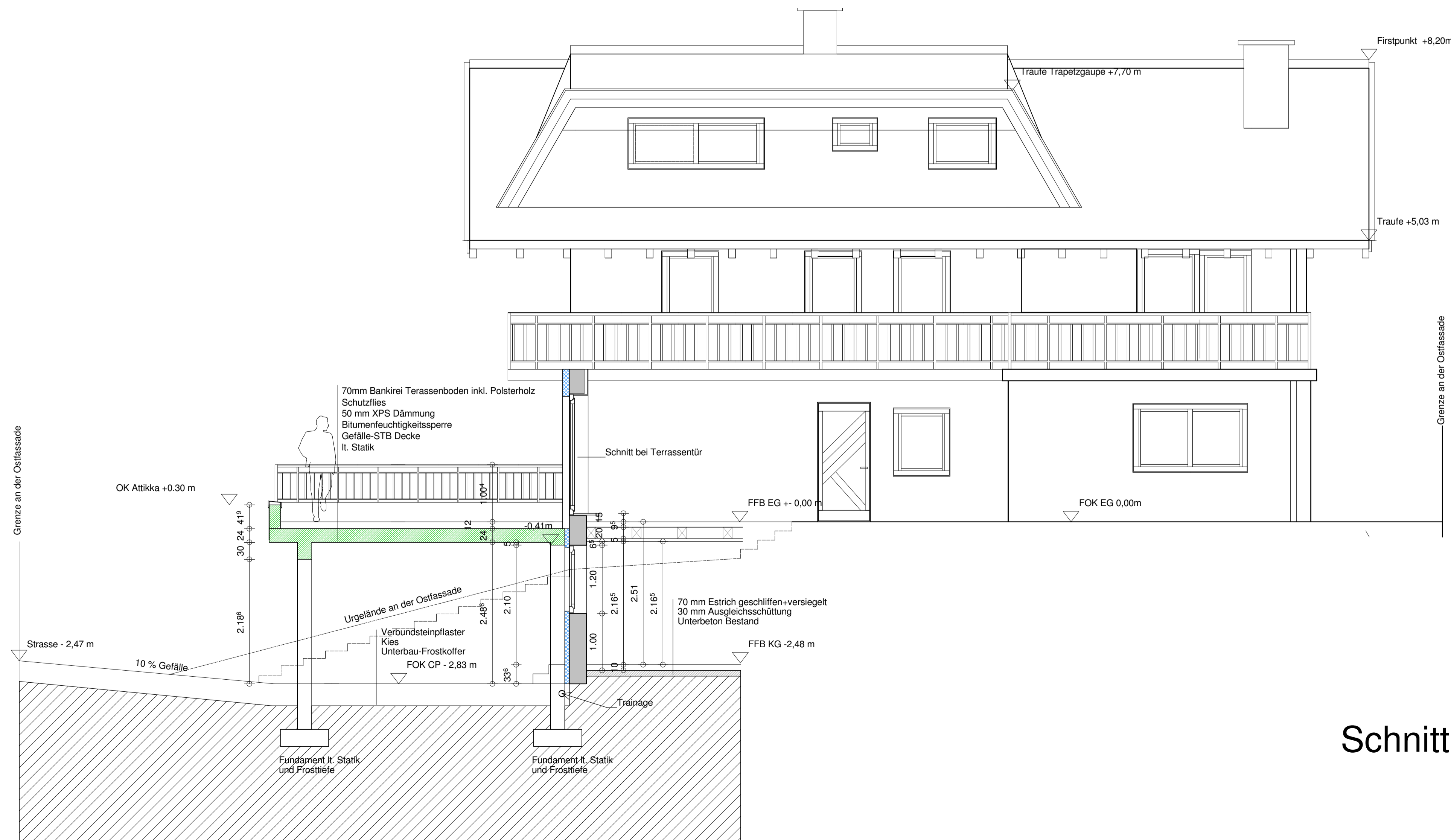
Schnitt A-A
